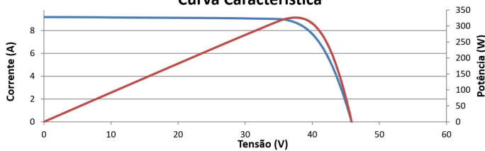
Curva Característica
